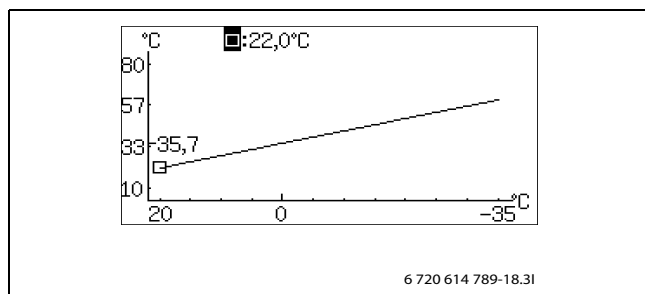
Fig. 22 Innstillingsvindu Varmekurve (radiator)
