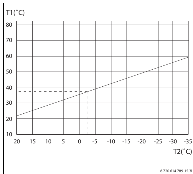
Fig. 20 Radiator
