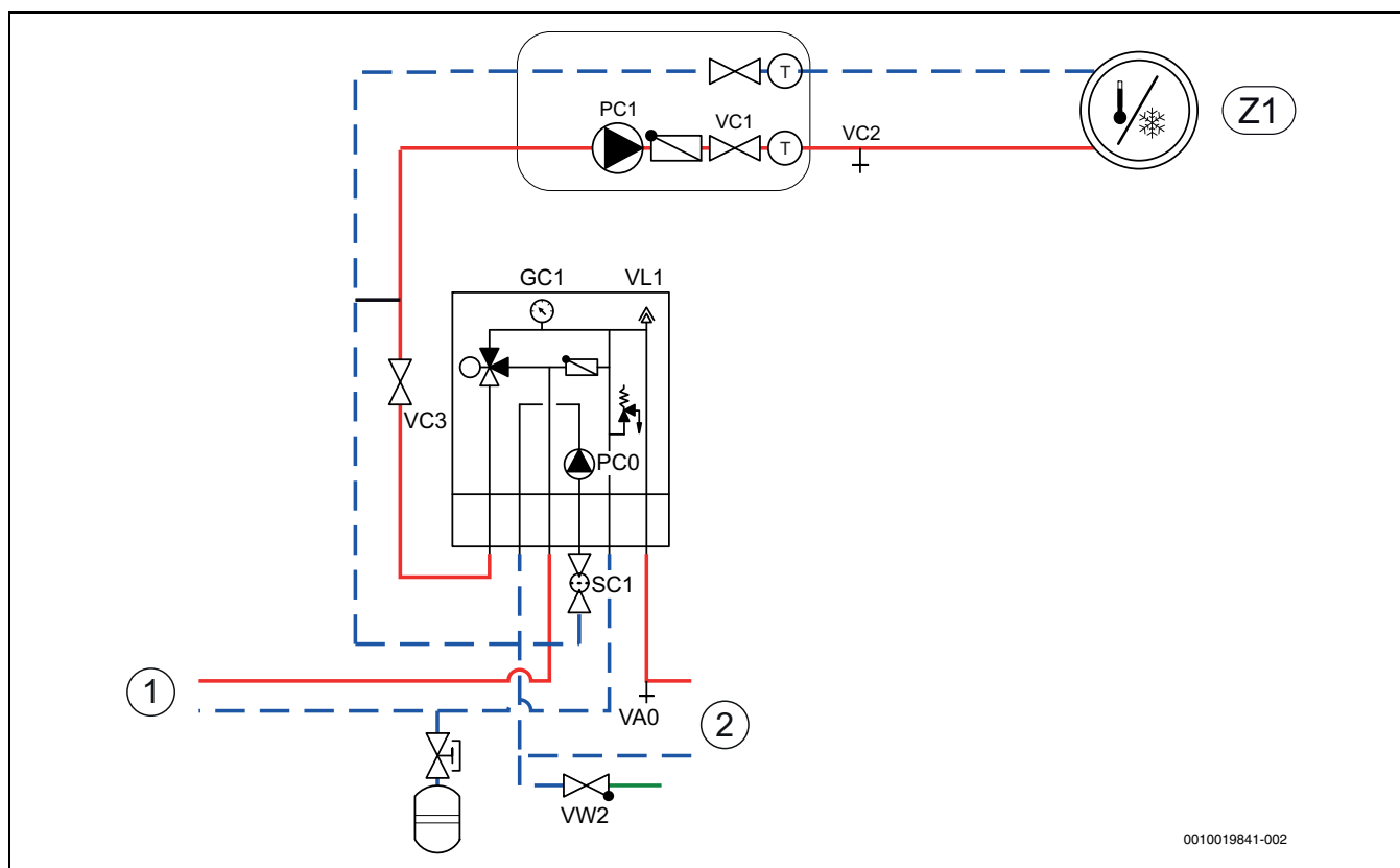
Fig. 9 Innvendig enhet med eksternt tilskudd og varmesystem
