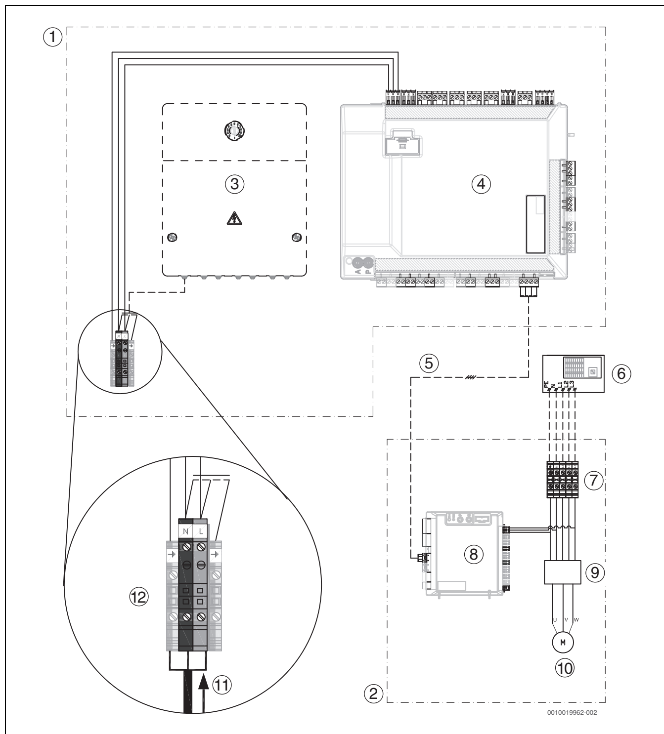
Fig. 36 Trefaset varmepumpe og innvendig enhet med eksternt tilskudd
