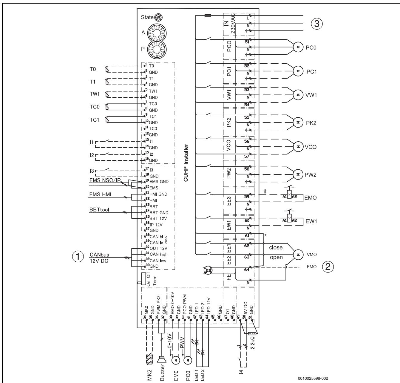
Fig. 37 Kablingsskjema installasjonsmodul for innvendig enhet med shuntventil for eksternt tilskudd
