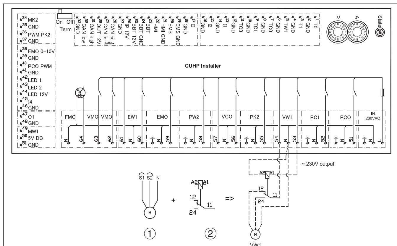
Fig. 40 Alternativ installasjon 3-veis-vekselventil
