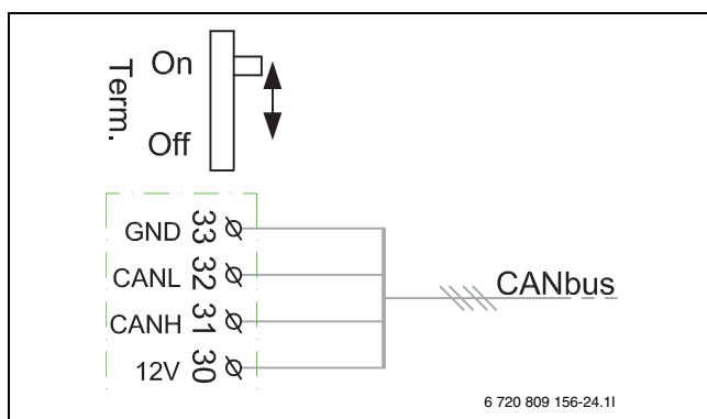
Fig. 10 CAN-BUS-terminering
