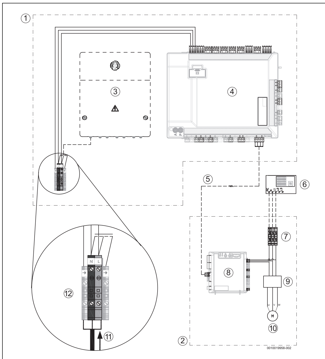
Fig. 35 Enfaset varmepumpe og innvendig enhet med eksternt tilskudd
