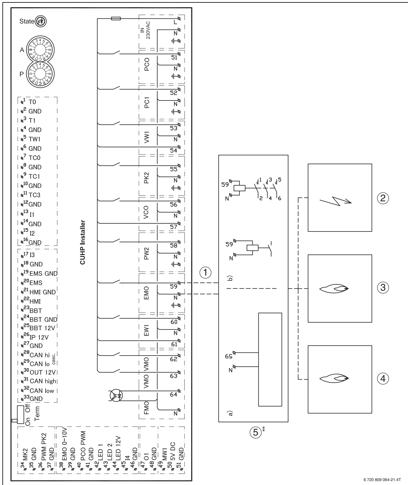
Fig. 38 Koblingsskjema for installasjonsmodul, start/stopp med eksternt tilskudd
