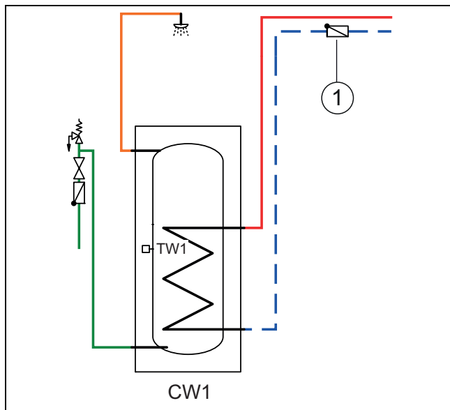
Fig. 24 Varmtvannsbereder
