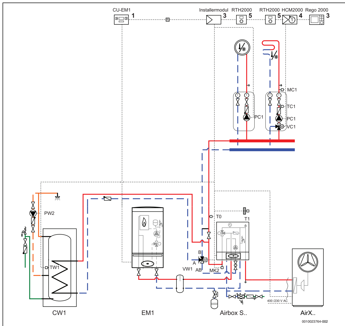
Fig. 33 Tilskudd med shunt med varmtvannsbereder
