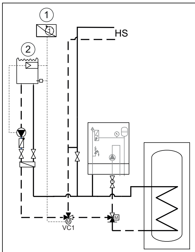
Fig. 29 Eksempelvisning for basseng-installasjon
