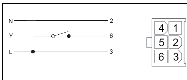
Fig. 28 Molex-støpsel
