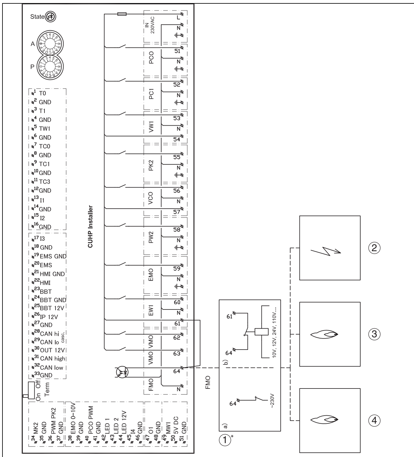
Fig. 39 Kablingsskjema for installasjonsmodul, alarm for eksternt tilskudd
