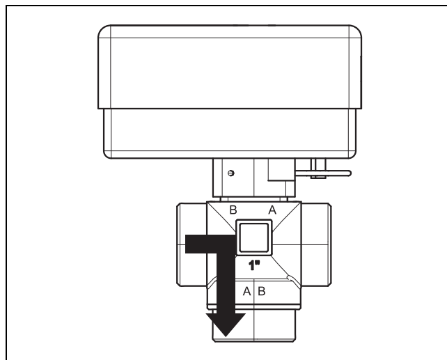
Fig. 27 Åpne kontakt, åpne tilkobling B
