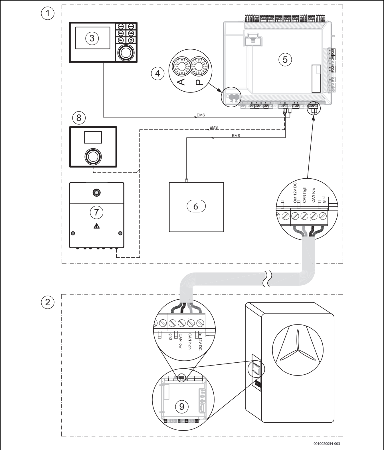
Fig. 34 Innvendig enhet med shuntventil for eksternt tilskudd – Oversikt CAN-/EMS-BUS
