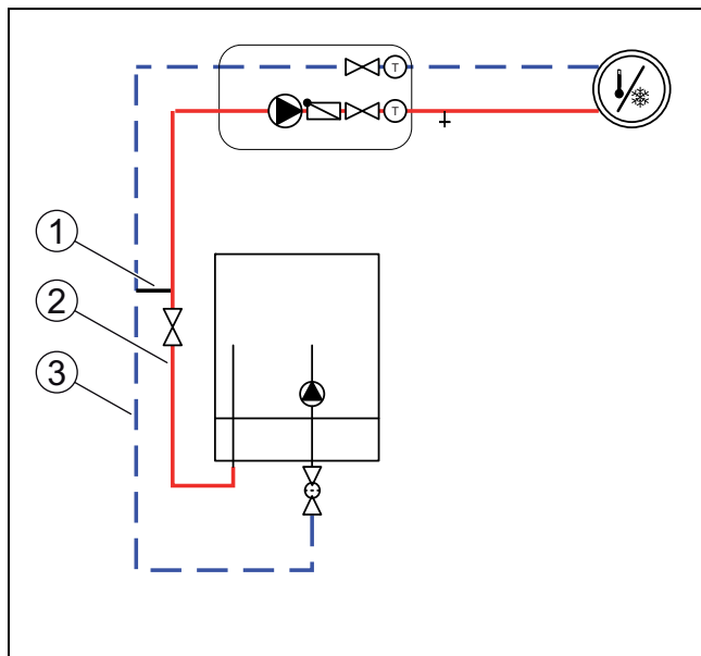
Fig. 31 Innvendig enhet med varmekrets og bypass
