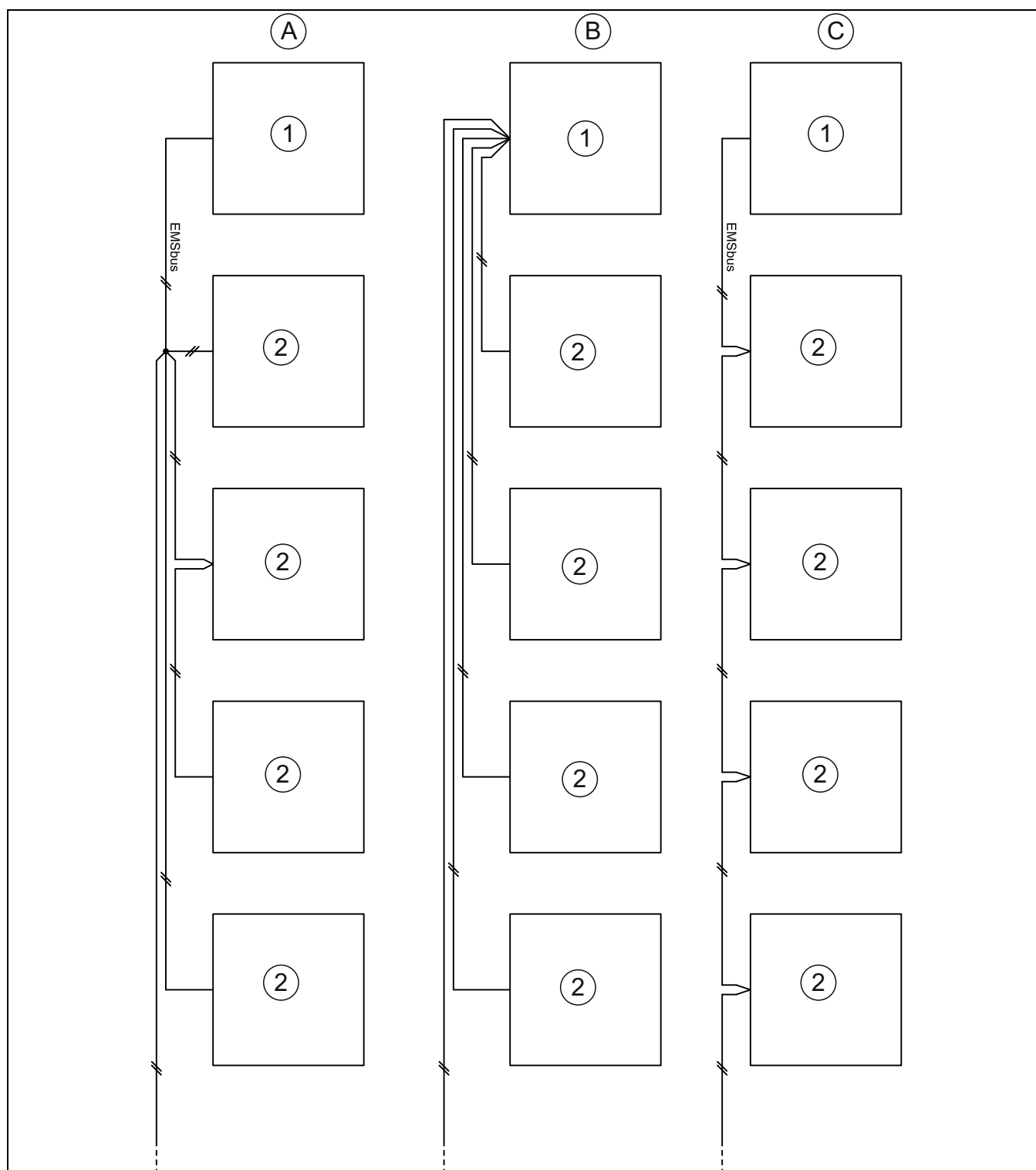
Fig. 15 Tilkoblingsalternativ for EMS-buss
