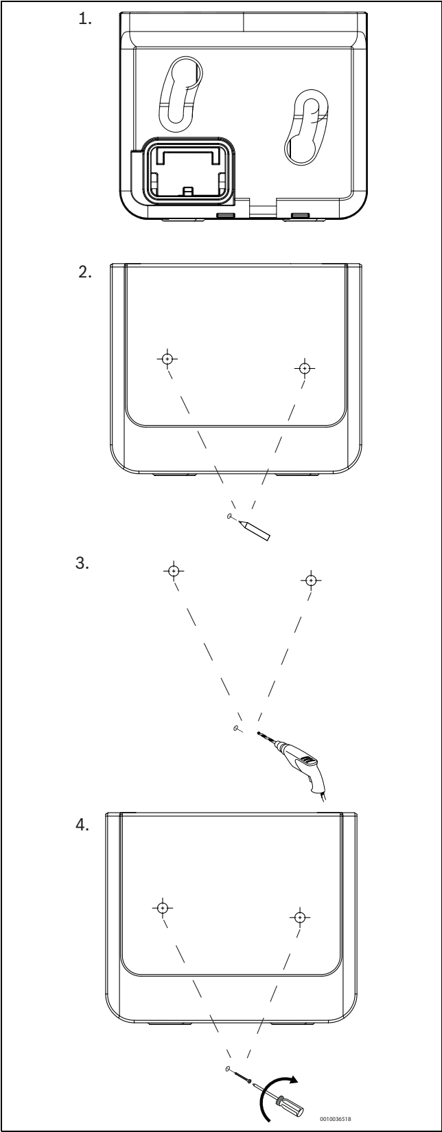
Fig. 19 Montering av holderen på vegg
