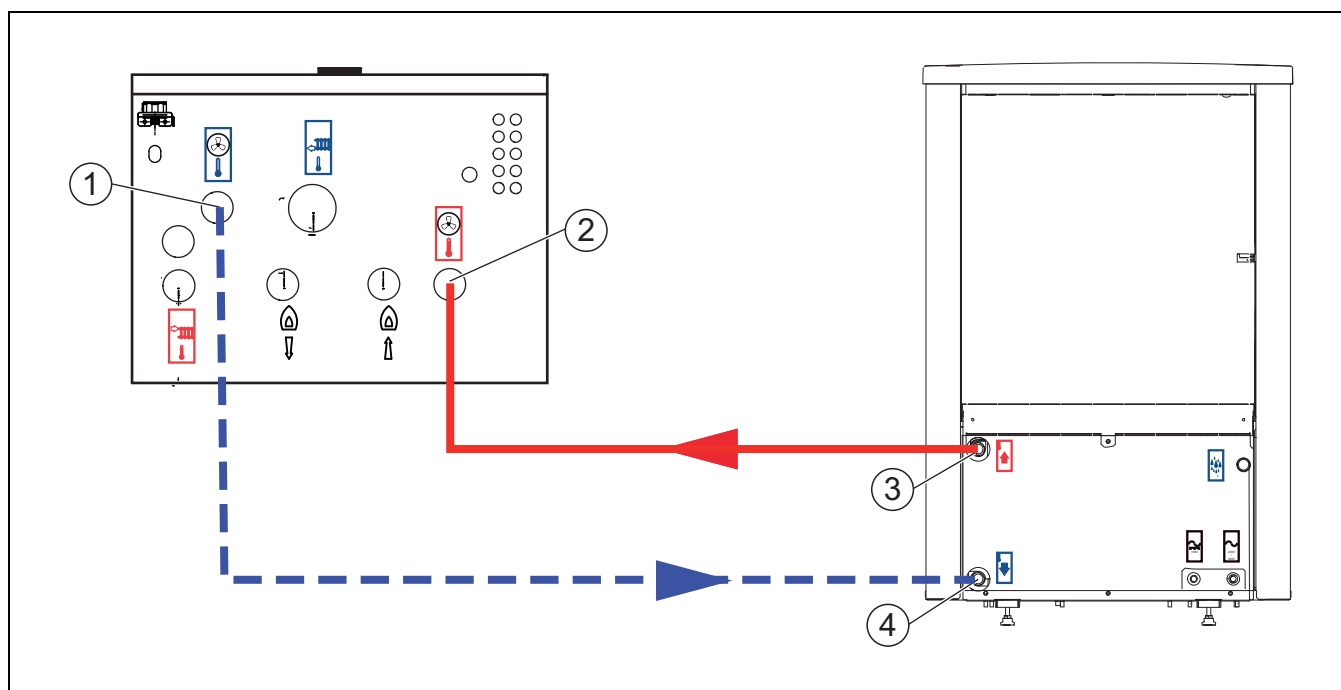
Fig. 7 Tilkobling fra den innvendige enheten til varmepumpen
