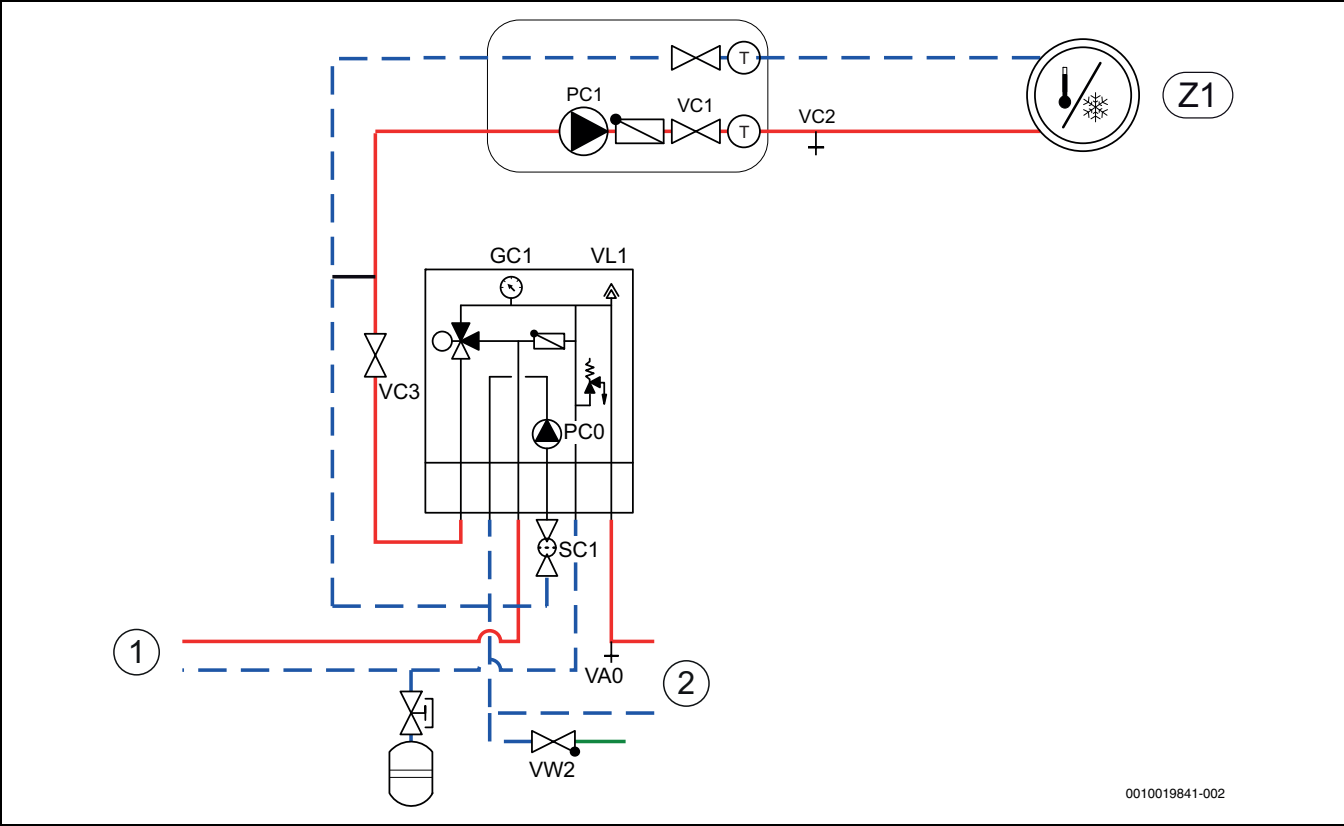
Fig. 21 Innvendig enhet med eksternt tilskudd og varmesystem
