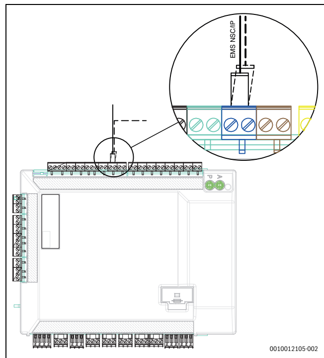
Fig. 23 EMS-tilkobling på installasjonsmodulen
