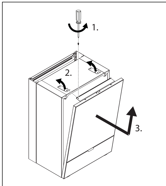
Fig. 6 Ta av frontplate
