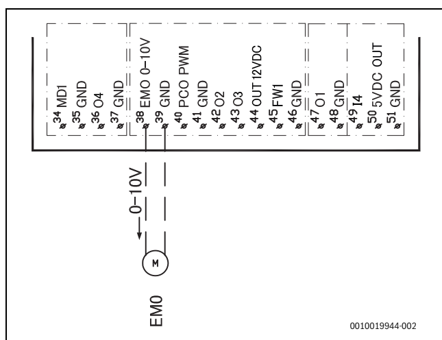
Fig. 14 0-til 10-V-aktivering for eksternt tilskudd
