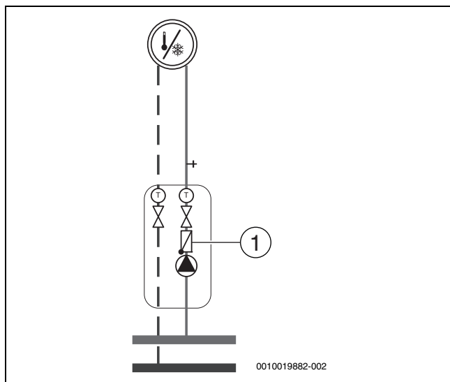
Fig. 32 Varmekrets
