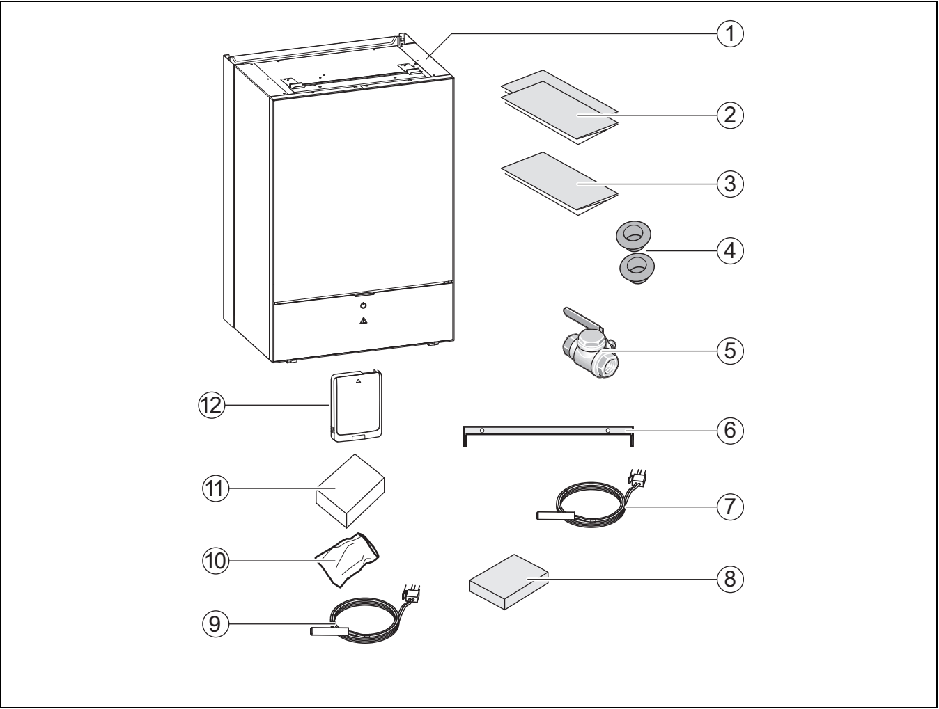
Fig. 2 Leveringsomfang
