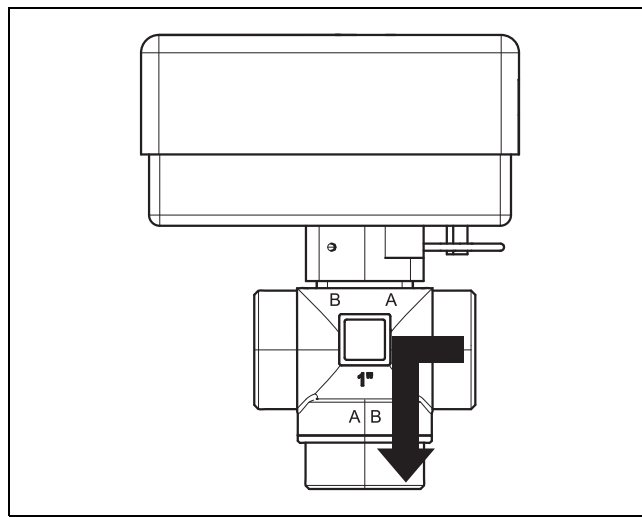
Fig. 26 Lukk kontakt, åpne tilkobling A
