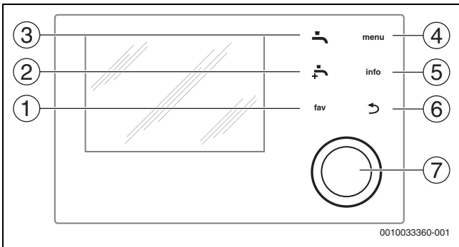
Fig. 4 Betjeningselementer
