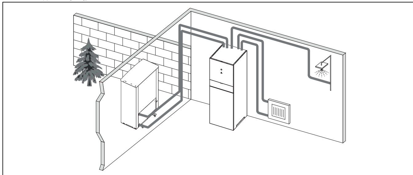
Fig. 3 Varmepumpe AirX 400, inneenhet AirModule E / AirModule S/W med integrert varmtvannsbereder og strømtilskudd
