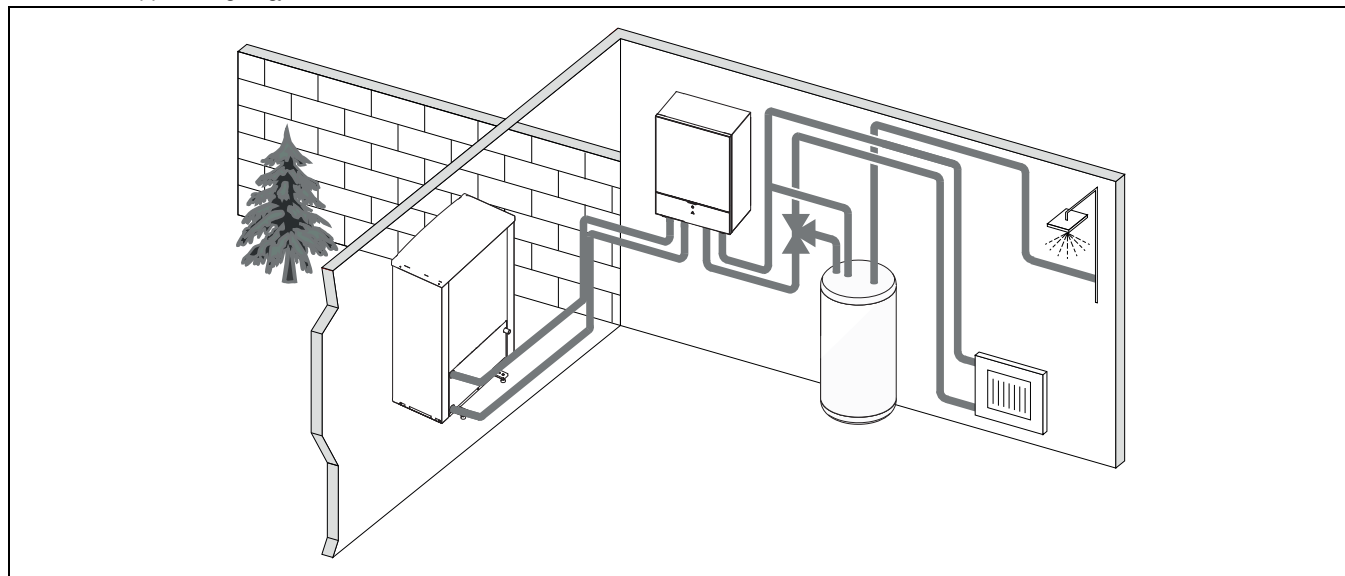
Fig. 3 Varmepumpe AirX 400, inneenhet Airbox E med strømtilskudd og ekstern varmtvannsbereder
